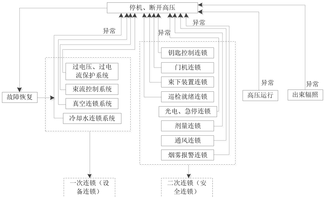
图 10-3 系统异常逻辑关系示意图
