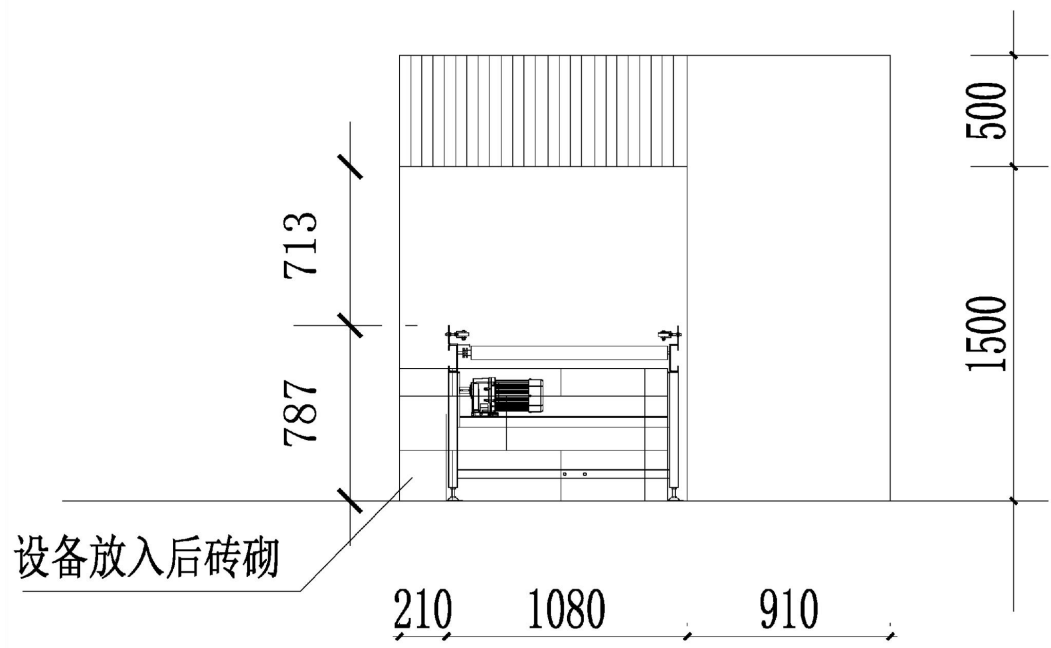
图 10-7 辐照室出入口剖面图（单位 mm）
