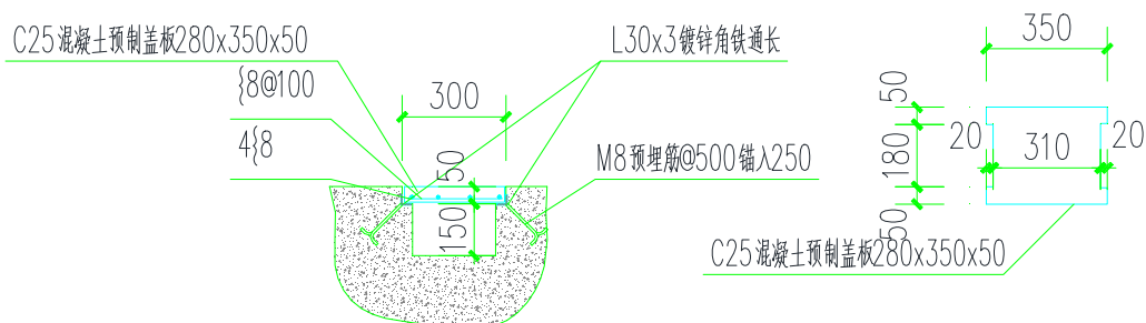
图 10-11 本项目电缆管线剖面示意图（单位 mm）
