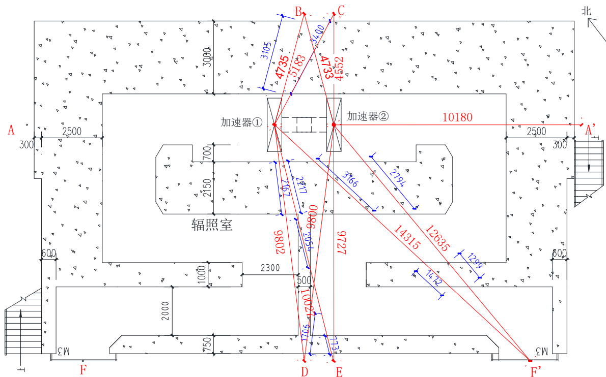
图 11-1 辐照室关注点
