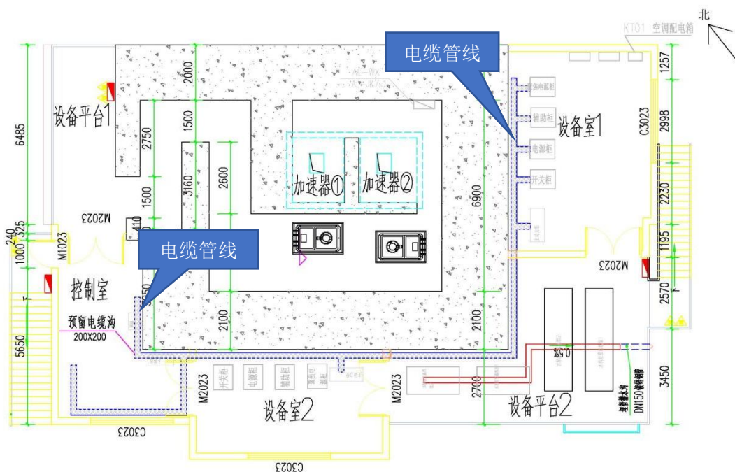
图10-9 主机室电缆管线的布设示意图（蓝色为电缆管线）（单位mm）
