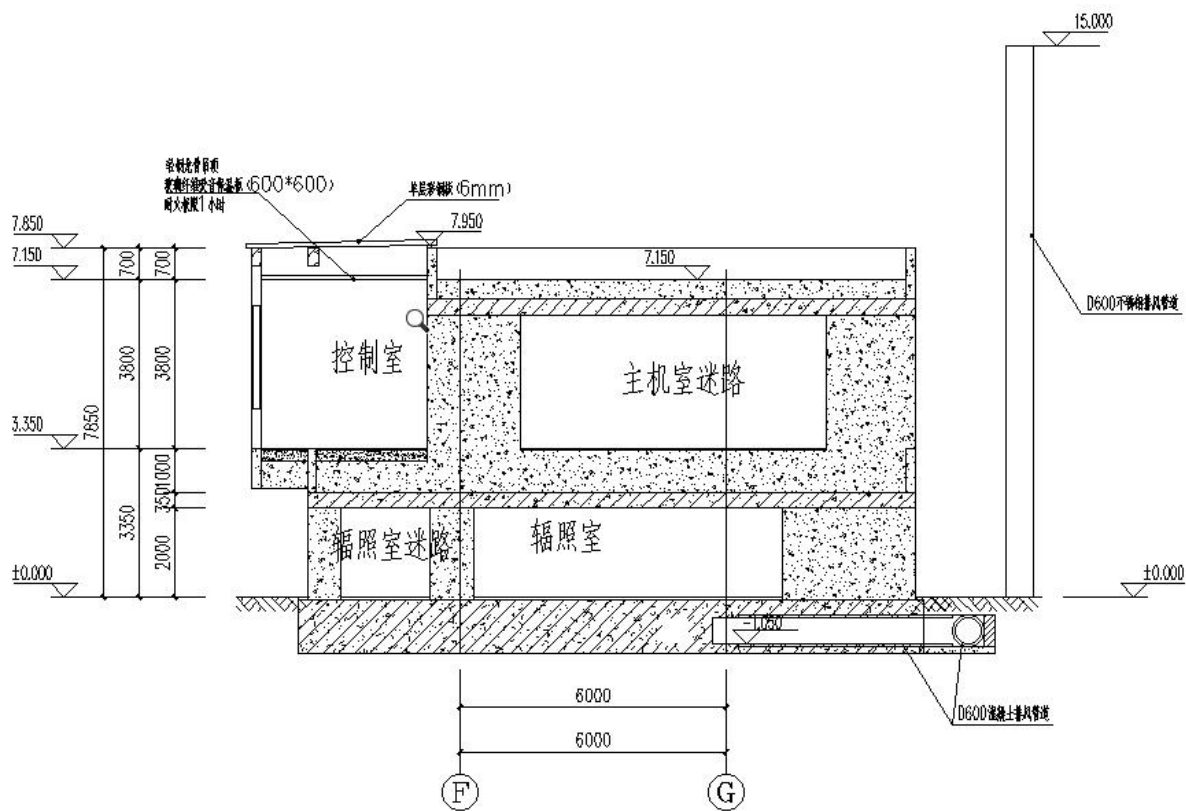
(e) 4-4 方向剖面图 (单位 mm)
