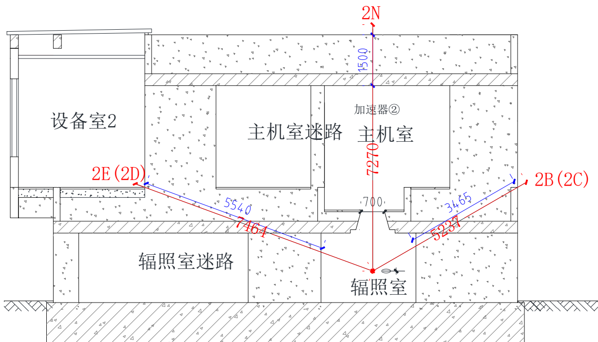
图 11-7 辐照室上方 3-3 剖面关注点图（加速器①上同）
