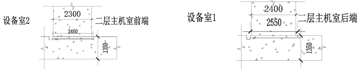
图 10-10 本项目电缆管线穿墙示意图（单位 mm）
