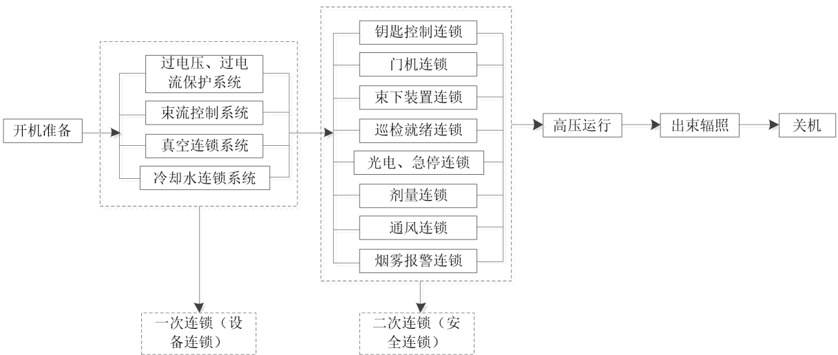
图 10-2 系统开机的安全联锁逻辑关系示意图
