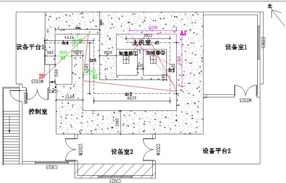
图 11-5 主机室散射路径示意图 1
