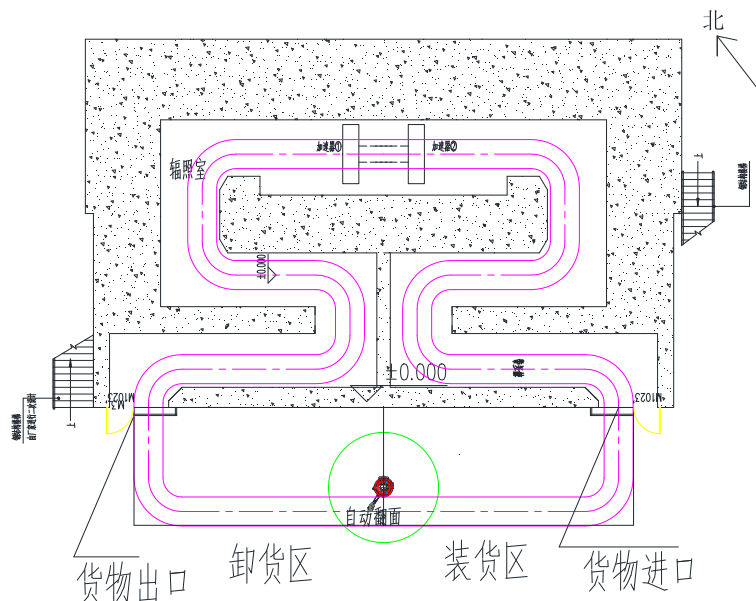
图 9-5 传送装置工作示意图
