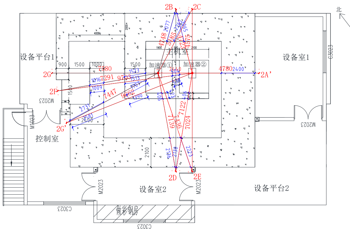
图 11-2 主机室关注点
