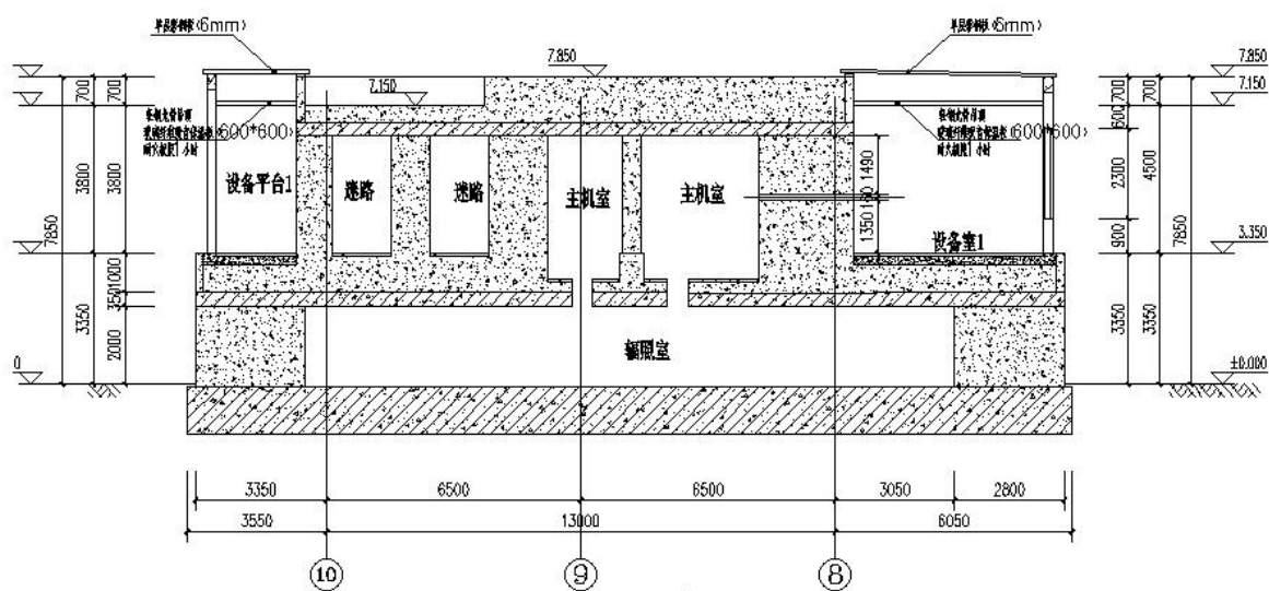
(c) 1-1 方向剖面图 (单位 mm)
