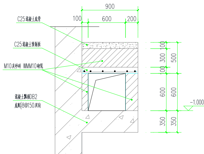
图 10-14 排风管剖面示意图
