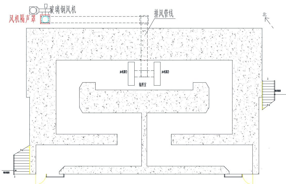
图 10-12 排风管道地埋设置平面示意图
