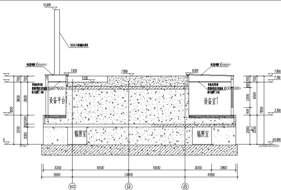
(d) 2-2 方向剖面图 (单位 mm)
