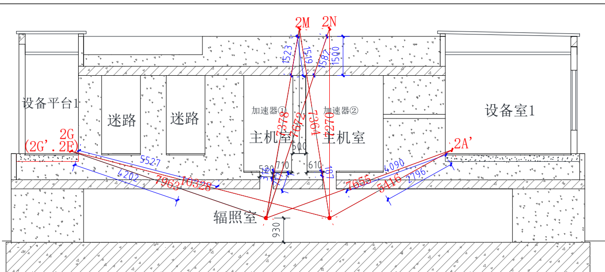
图 11-6 辐照室上方 1-1 剖面关注点图
