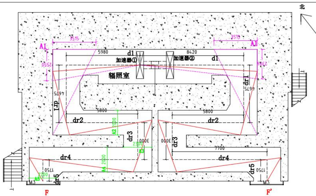
图 11-3 辐照室散射路径示意图 1
