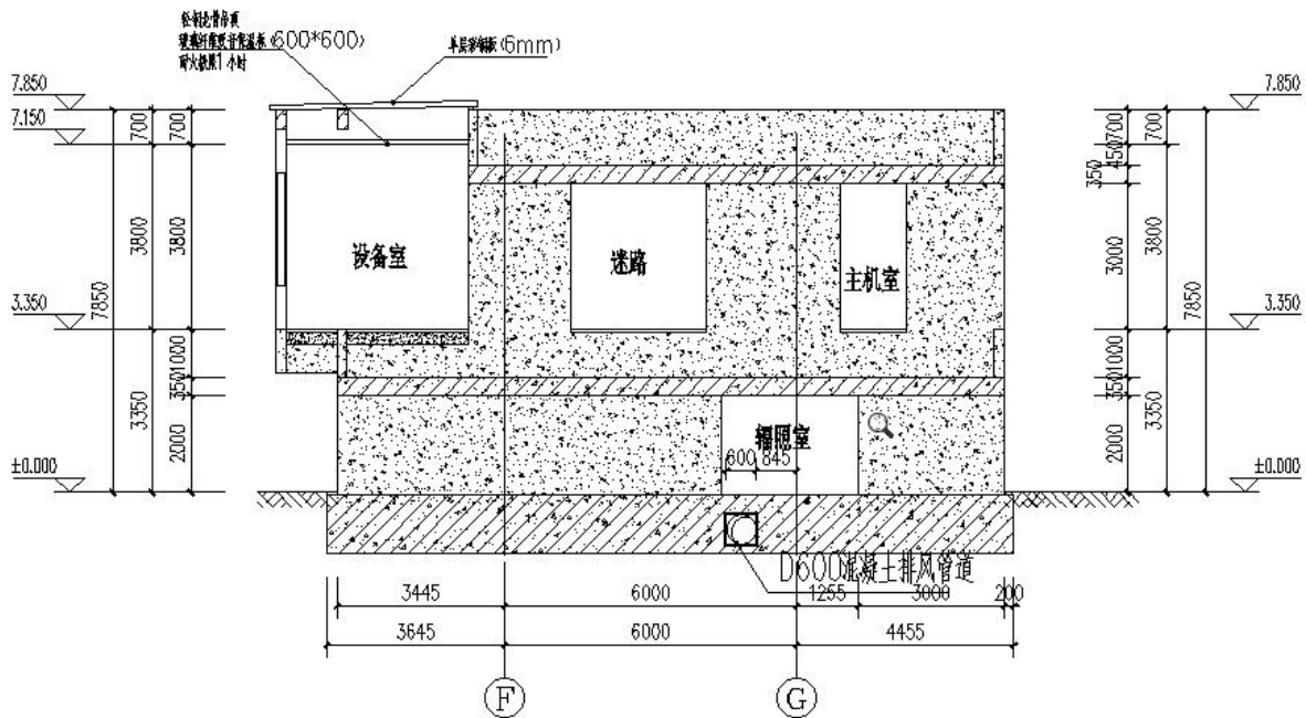
图 10-13 排风管道设置位置示意图
