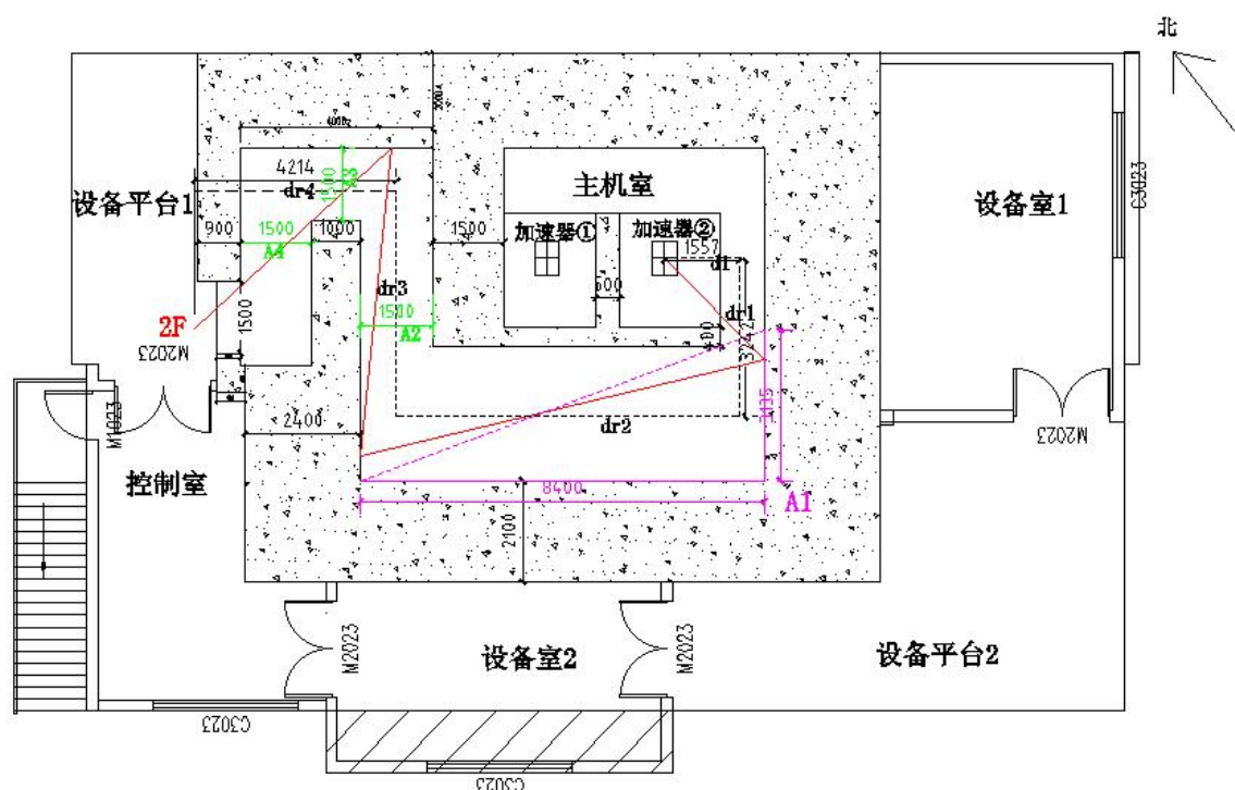
图 11-6 主机室散射路径示意图 2
