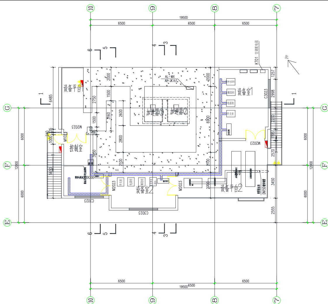
(b) 主机室平面布置图 (单位 mm)
