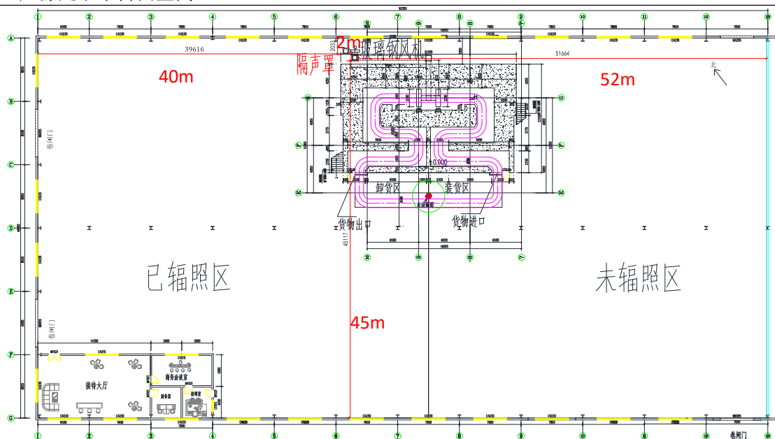
图 11-10 噪声边界示意图
